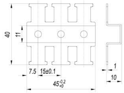
绑线板尺寸图
