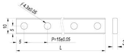
ACR10 导轨尺寸图
