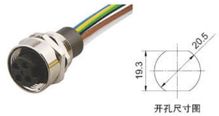
开孔尺寸图
