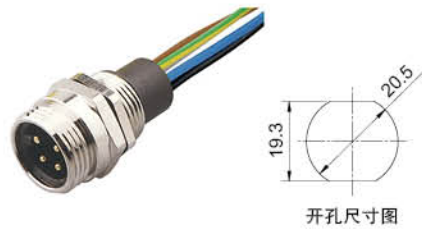
开孔尺寸图
