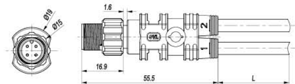
Y型线 Y-distributor
